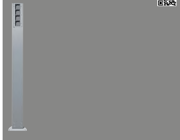
Gira Energiesäule mit 4 Leereinheiten Höhe 1600 mm
